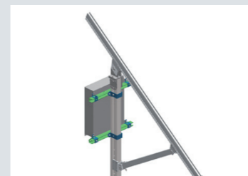
ソーラーテラスII-A (シングルサポート) 接続箱取付け用ブラケット
